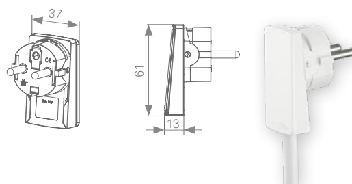
PlugMini Fix
